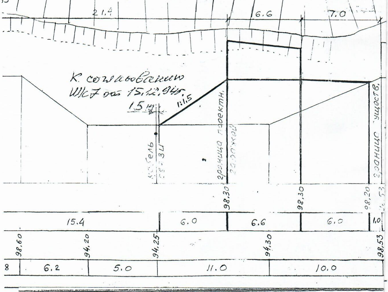
Поперечный профиль на ПК 3+00 масштаб 1:200
