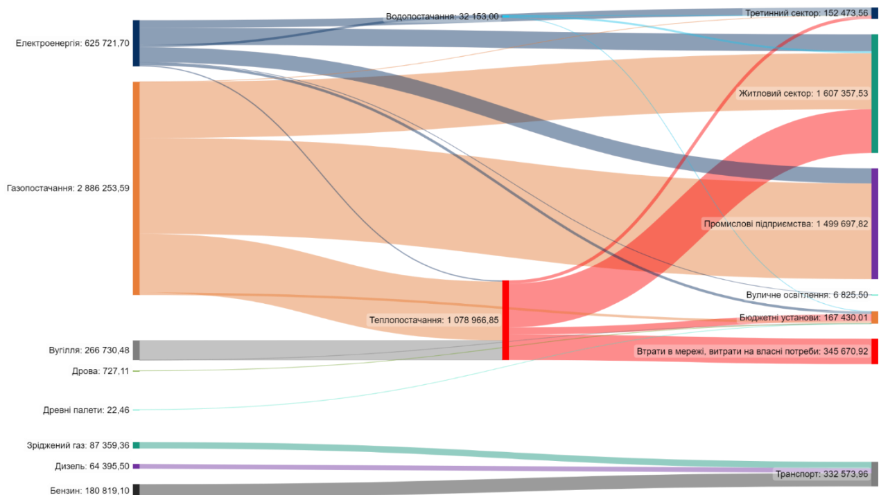
Рис. 3.1. Енергетичний баланс громади (діаграма Сенкі)
