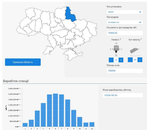
Рис. 1.10. Розрахунок теоретичної потужності СЕС згідно із визначеною площею 4
