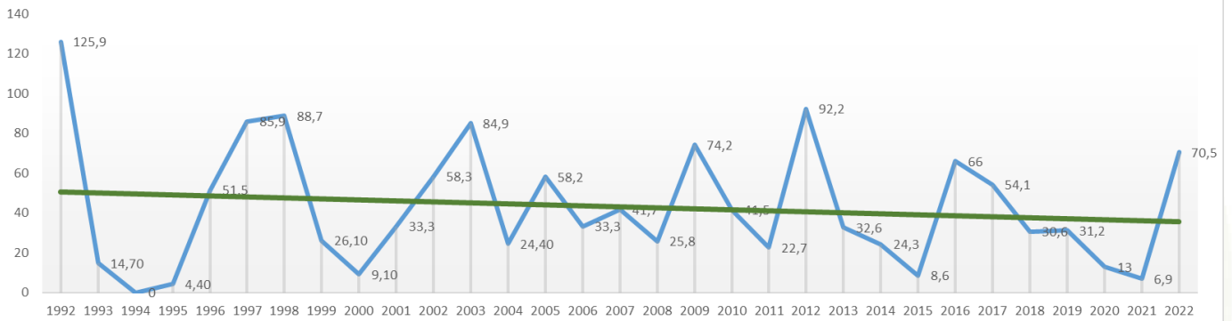
Кількість опадів за жовтень, мм
