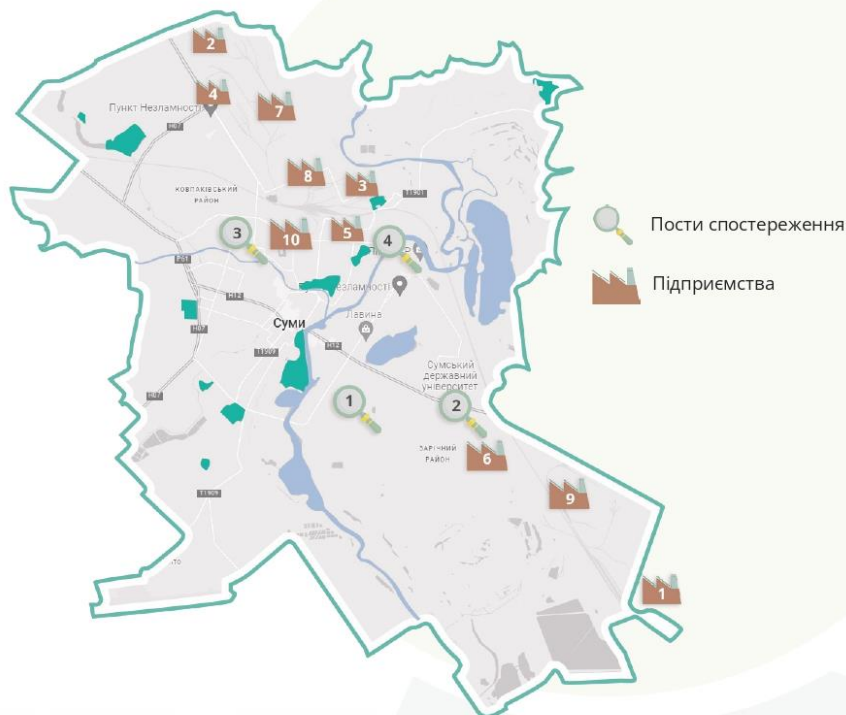
Зобр. 1 Розміщення основних стаціонарних джерел викидів та пунктів спостереження за станом атмосферного повітря у м. Суми
