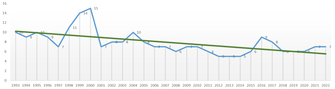
Максимально разова концентрація оксиду вуглецю, мг/м 3
