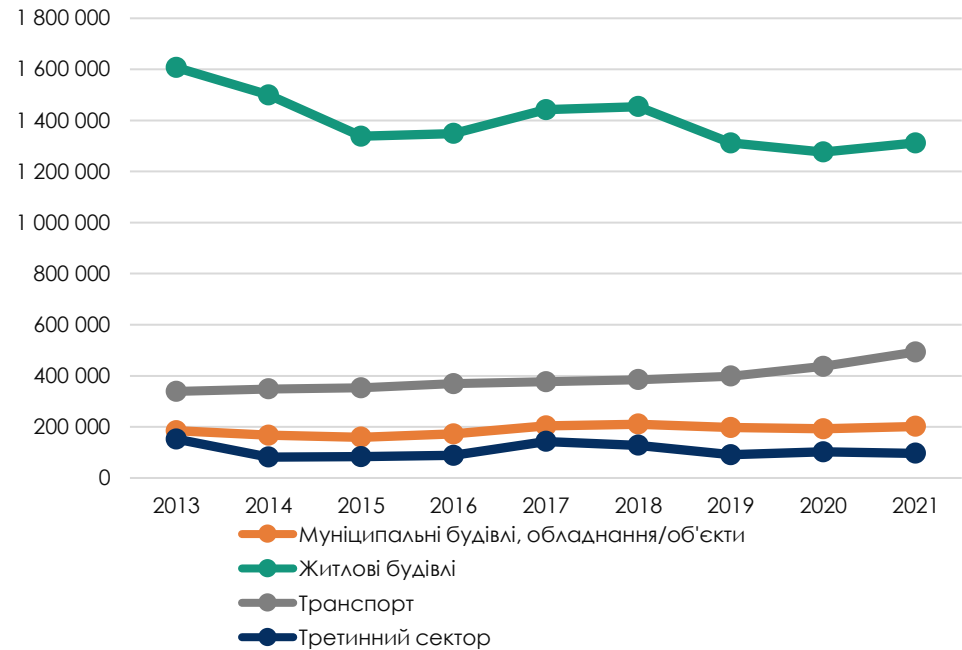
Рис. 3.7. Динаміка споживання енергоресурсів за 2013-2021 роки, МВт*год
