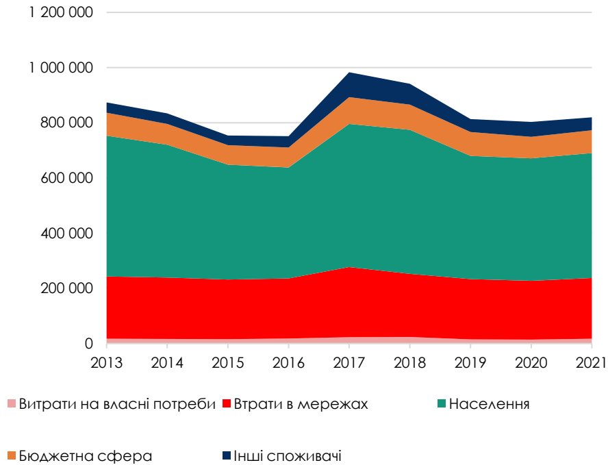
Рис. 2.5. Виробництво, втрати та споживання теплової енергії, Гкал
