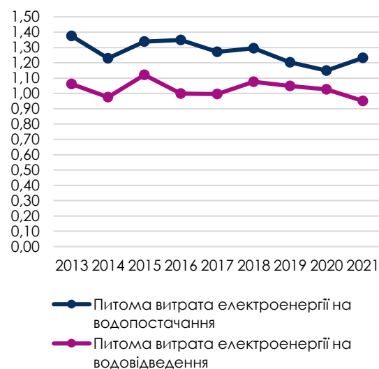
Рис. 2.16. Питомі витрати електроенергії на водопостачання та водовідведення, кВт*год/м 3
