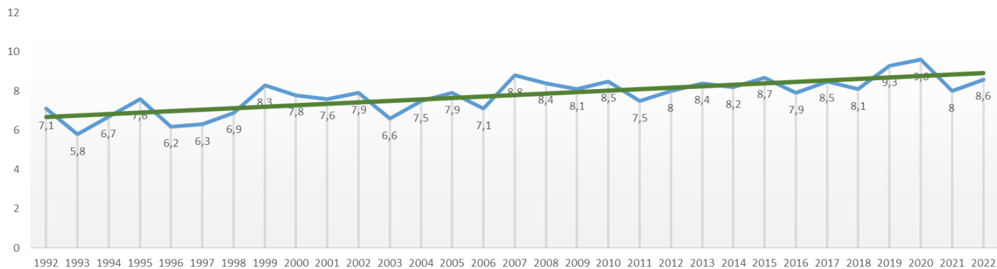
Середньорічна температура повітря, 0С
