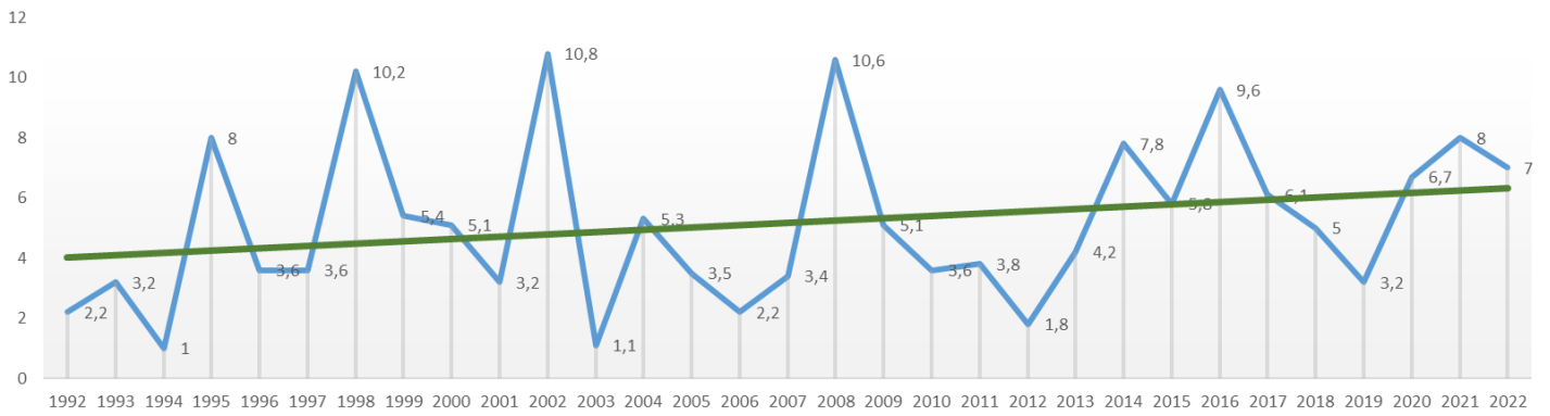
Максимальна температура повітря за лютий, ОС
