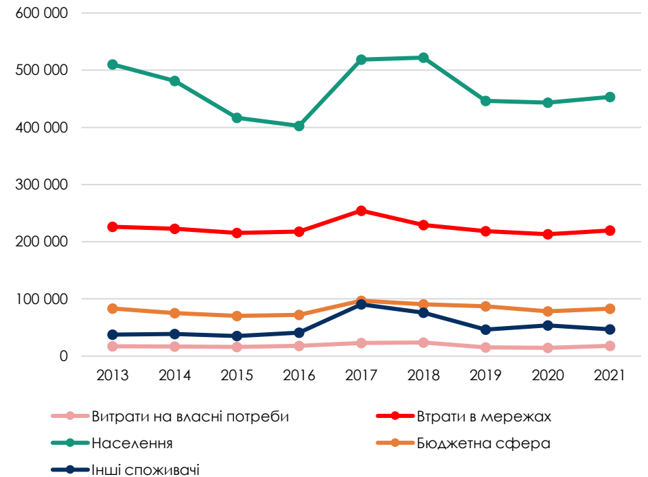
Рис. 2.6. Виробництво, втрати та споживання теплової енергії, Гкал
