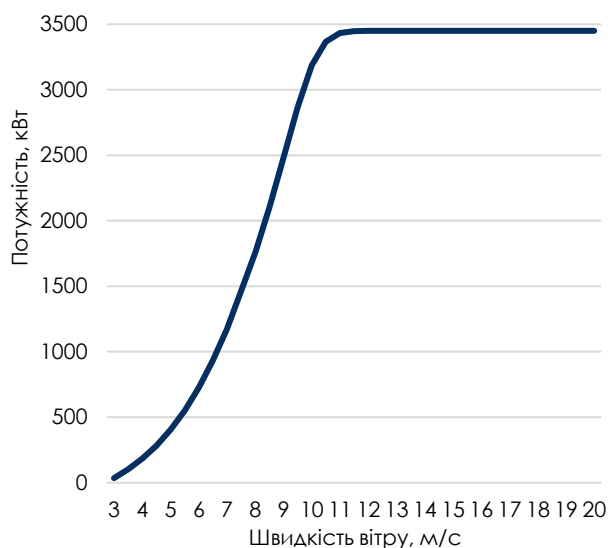
Рис. 1.11. Крива потужності віротурбіни Vestas V126-3.45.
