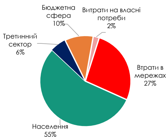
Рис. 2.4. Загальний річний баланс теплової енергії у питомих показниках за 2021 рік
